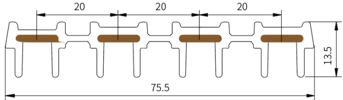
Чертёж (в масштабе 1:1)
