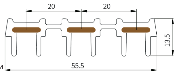
Чертёж (в масштабе 1:1)
