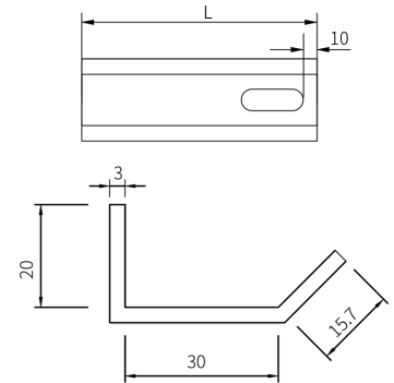
Специальный кронштейн AN
